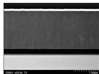
実物の断面観察像（透過電子顕微鏡像）
